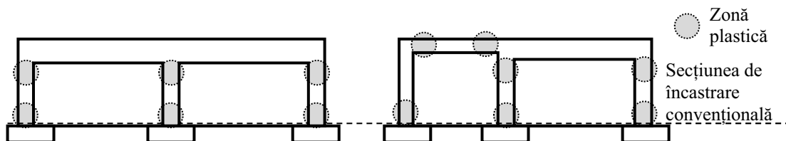
Figura 3.12 Reprezentare exemplificativă a unui mecanism plastic optim: poziționarea zonelor plastice pentru o structură în cadre cu un singur nivel, cu deschideri mari
