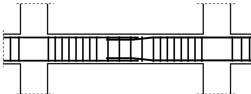
Figura 6.14 Detaliu de principiu cu suprapunerea armăturilor într-o grindă
