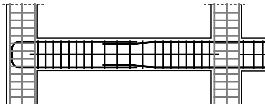
Figura 6.18 Detaliu de principiu cu armarea longitudinală a stâlpului care traversează nodul
