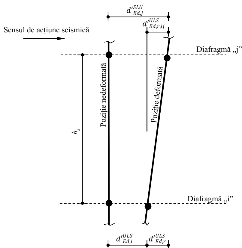
Figura 3.17 Reprezentare exemplificativă: calculul deplasării relative de nivel pentru o structură etajată
