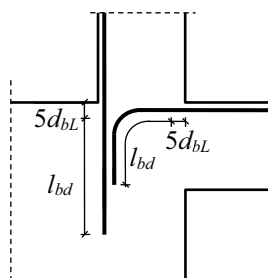
Figura 6.15 Reprezentare exemplificativă privind ancorarea armăturilor din zonele critice ale grinzilor și stâlpilor
