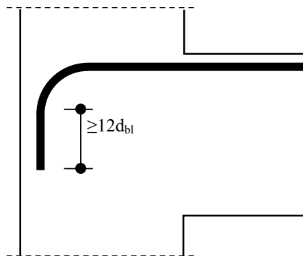
Figura 6.16 Lungimea minimă a ciocului pentru armăturile longitudinale din grinzi
