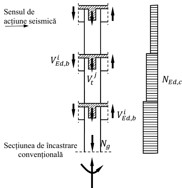
Figura 4.3 Calculul valorilor de proiectare ale forței axiale în stâlpi
