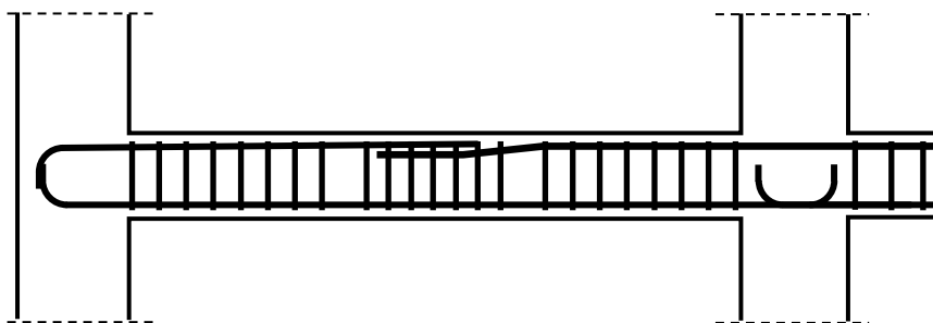
Figura 6.17 Detaliu de principiu cu ancorarea barelor longitudinale ale grinzilor în nod
