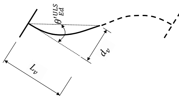
Figura 3.18 Rotirea de bară determinată prin calcul static liniar în gruparea seismică
