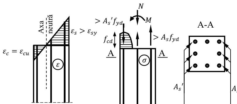
Figura 3.14 Reprezentare exemplificativă: starea de eforturi unitare și de deformații specifice pe secțiune corespunzătoare cedării din încovoiere pentru un stâlp
