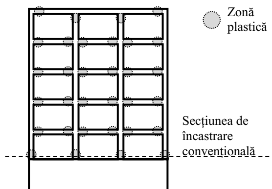
Figura 3.10 Reprezentare exemplificativă a unui mecanism plastic optim: poziționarea zonelor plastice pentru o structură în cadre multietajată
