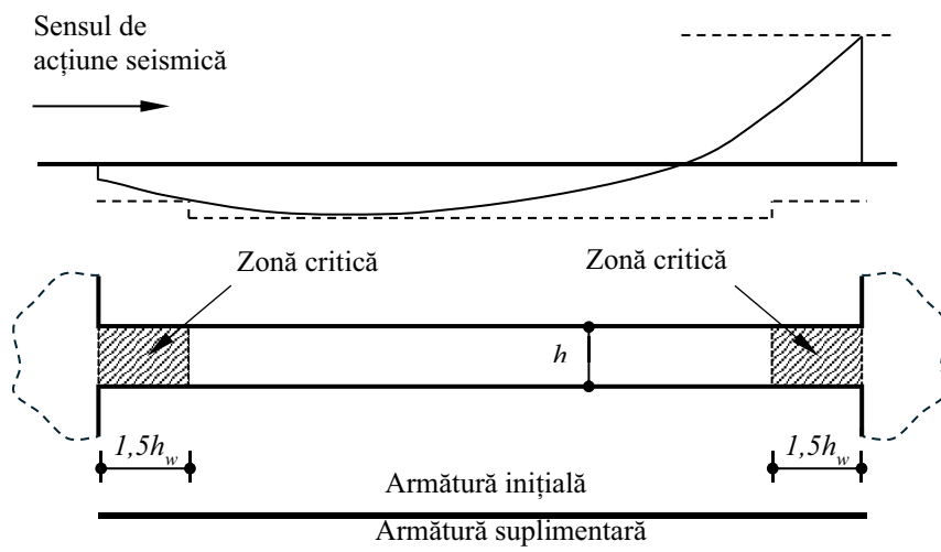
Figura 3.9 Reprezentare exemplificativă cu dirijarea zonelor plastice către capetele grinzii prin suplimentarea locală a armăturii longitudinale
