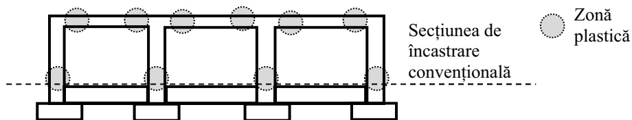
Figura 3.11 Reprezentare exemplificativă a unui mecanism plastic optim: poziționarea zonelor plastice pentru o structură în cadre cu un singur nivel, cu deschideri mici
