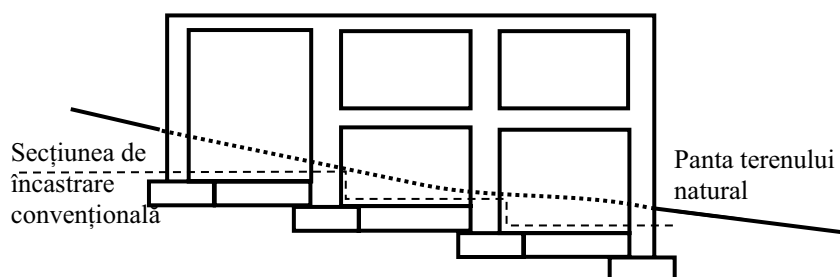
Figura 3.4 Reprezentare exemplificativă privind poziționarea secțiunii de încastrare convențională pentru o clădire în cadre de beton armat amplasată pe teren în pantă, cu cota de fundare variabilă
