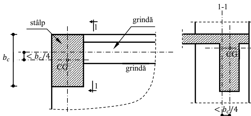
Figura 6.2 Représentare exemplificativă privind limitarea excentricității orizontale grindă-stâlp pentru clasa de ductilitate DCH
