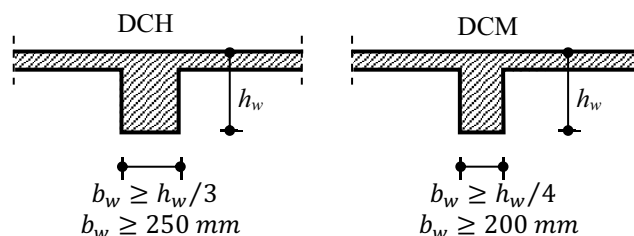
Figura 6.1 Lățimea minimă a secțiunii transversale a grinzilor
