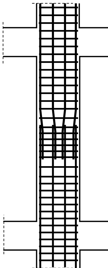
Figura 6.19 Detaliu de principiu cu ancorarea și suprapunerea armăturilor la jumătatea înălțimii libere a stâlpului
