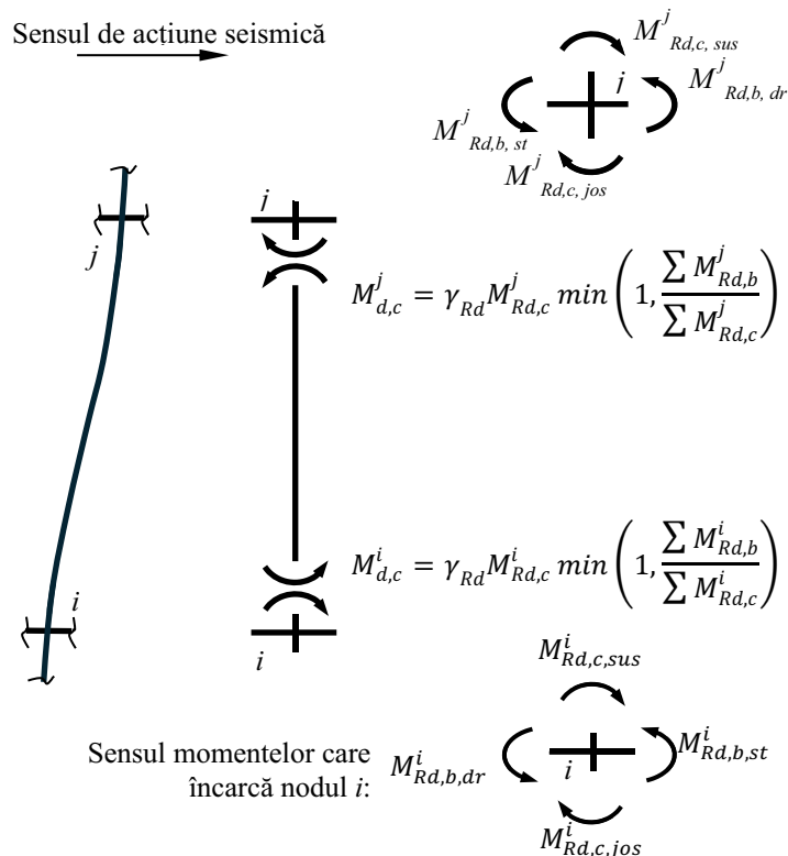
Figura 4.4 Determinarea valorilor momentelor încovoietoare maxime care încarcă stâlpul la capete, etaj curent
