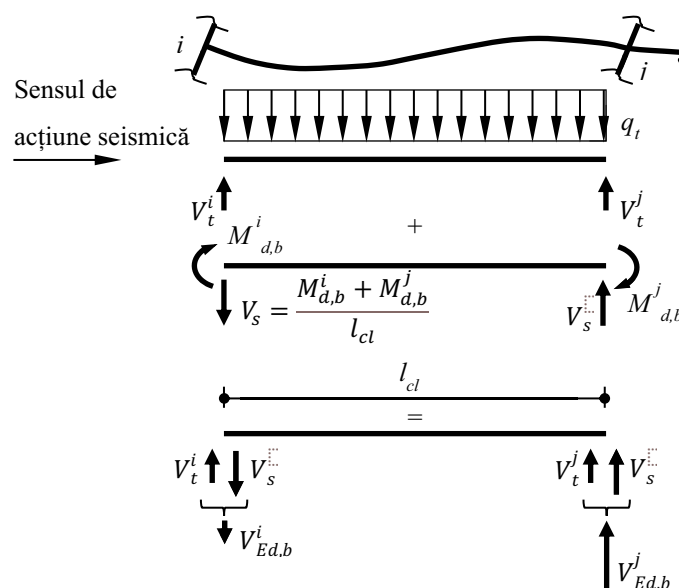
Figura 4.2 Schema de calcul a valorii de proiectare a forței tăietoare din grindă, când zonele plastice se formează la capetele acestora
