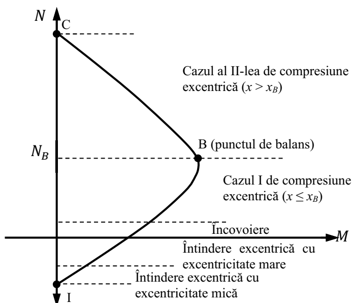
Figura 3.15 Curba limită de interacțiune M-N
