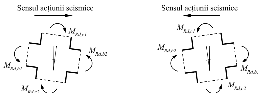
Figura 3.16 Sensul considerat al momentelor în verificarea condiției de la (3.8) pentru un nod grindă-stâlp
