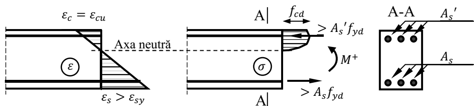
Figura 3.13 Reprezentare exemplificativă: starea de eforturi unitare și de deformații specifice pe secțiune corespunzătoare cedării din încovoiere pentru o grindă
