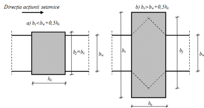
Figura 5.2 Stabilirea lăţimii de proiectare a nodului
