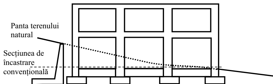
Figura 3.5 Reprezentare exemplificativă privind poziționarea secțiunii de încastrare convențională pentru o clădire în cadre de beton armat amplasată pe teren în pantă, cu cotă unică de fundare
