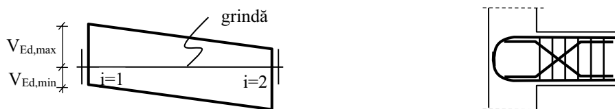
Figura 6.7 Reprezentare informativă privind semnificația mărimilor V_{Ed,max} și V_{Ed,min} și modul de dispunere a armăturii înclinate în zona critică a grinzilor
