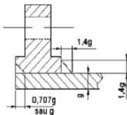
4. FLANȘĂ PLATĂ PT. SUDAT
