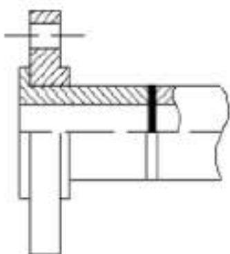
3. FLANȘĂ PLATĂ PT. SUDAT
