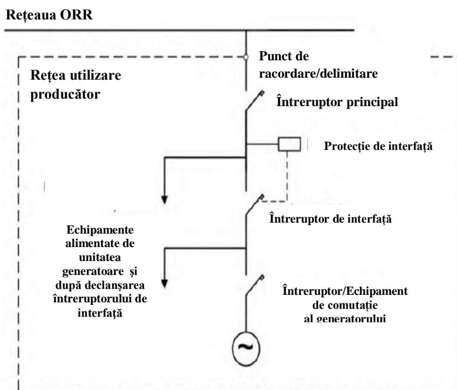
Figure 2 – Fig. 1. Exemplu de unități generatoare racordate la rețeaua operatorului de distribuție (schemă de principiu a echipamentelor de comutație/întreruptoare)
