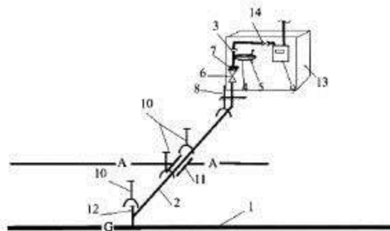
Fig. 9 Branșament de gaze naturale executat din oțel (exemplu)
