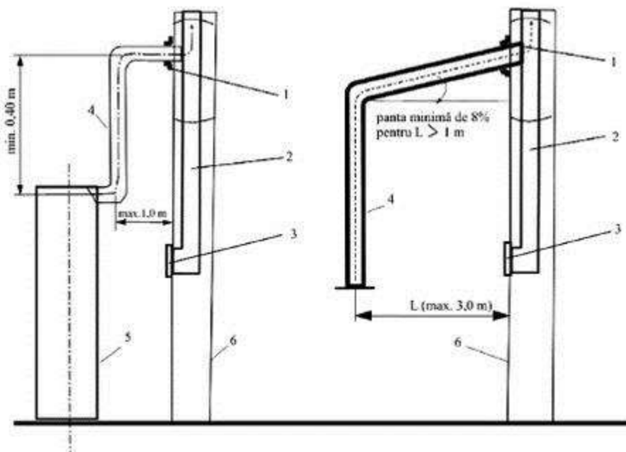
Fig. 13 Racordarea la coș de fum cu burlane
