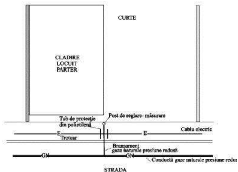
Fig. 8 Exemplu de alimentare a unui imobil
